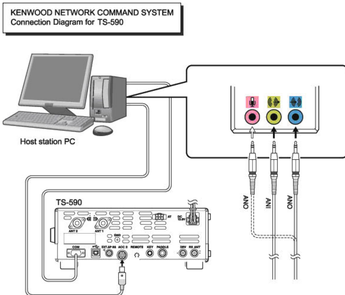
図：4.2.2 音声ケーブルの接続
