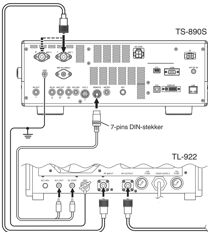
REMOTE Connector (Weergave van Achterpaneel)
