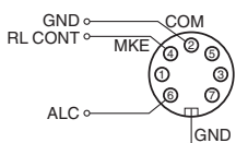
REMOTE Connector (Weergave van Achterpaneel)
