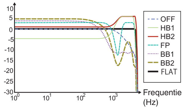
RX-karakteristiekcurve
