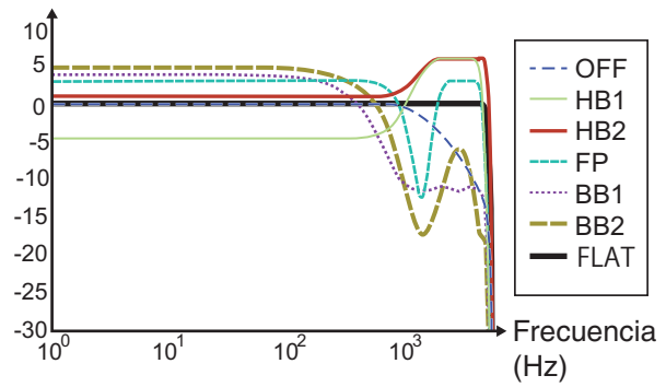
Curva característica de RX
