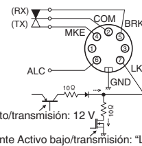
Conector REMOTE (vista del panel trasero)
