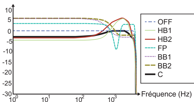
Courbe caractéristique TX
