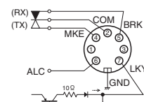
Connecteur REMOTE (vue depuis le panneau arrière)
