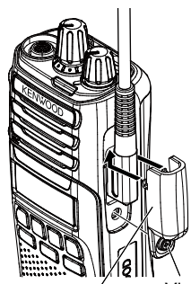
Support de verrouillage du haut- parleur/ microphone Vis
