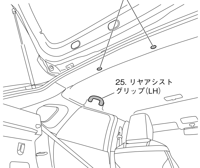
24. ルーフライニングクリップ
